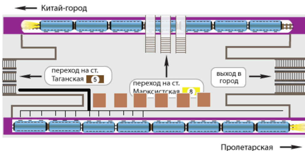
Рис. 1. Схема станции метро «Таганская»
